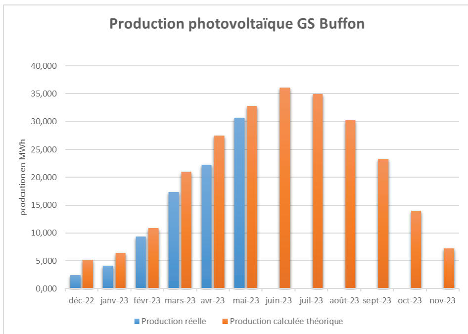
Figure 1 - On constate un bon accord entre la production attendue et la production effectivement accomplie sur l'école Buffon.
