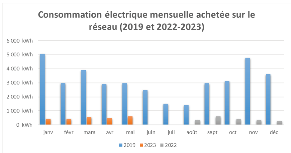
Figure 2 - On constate la réduction considérable (-80-90%) d'électricité achetée sur le réseau Enedis pour l'école Buffon, qui subvient à l'essentiel de ses besoins en électricité, même en hiver. En dehors de l'hiver, l'école Buffon produit un tel surplus (plus de 10 fois ses propres besoins !) qu'elle peut partager ce surplus avec les autres bâtiments de la Ville de Dijon situés dans le quartier Fontaine d'Ouche.
