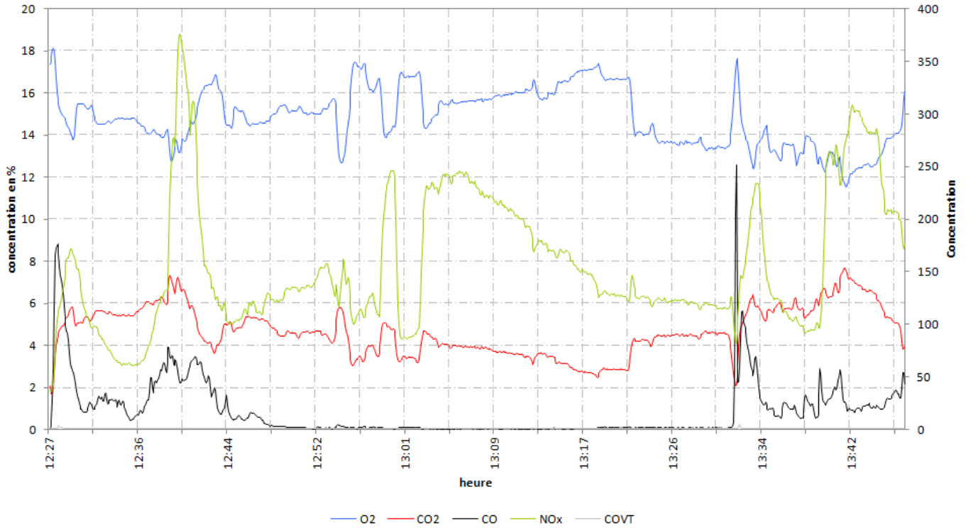
Courbes gaz - Crématorium de Dijon Appareil de crémations Le jeudi 13 février 2020 de 12:28 à 13:48
